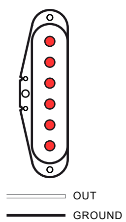
STANDARD STRATO
